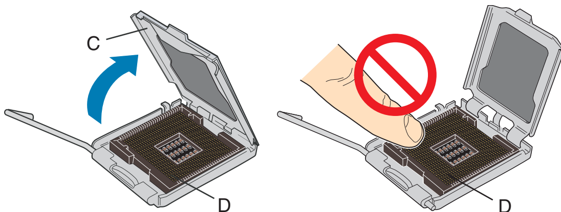
图 7. 抬起压板
