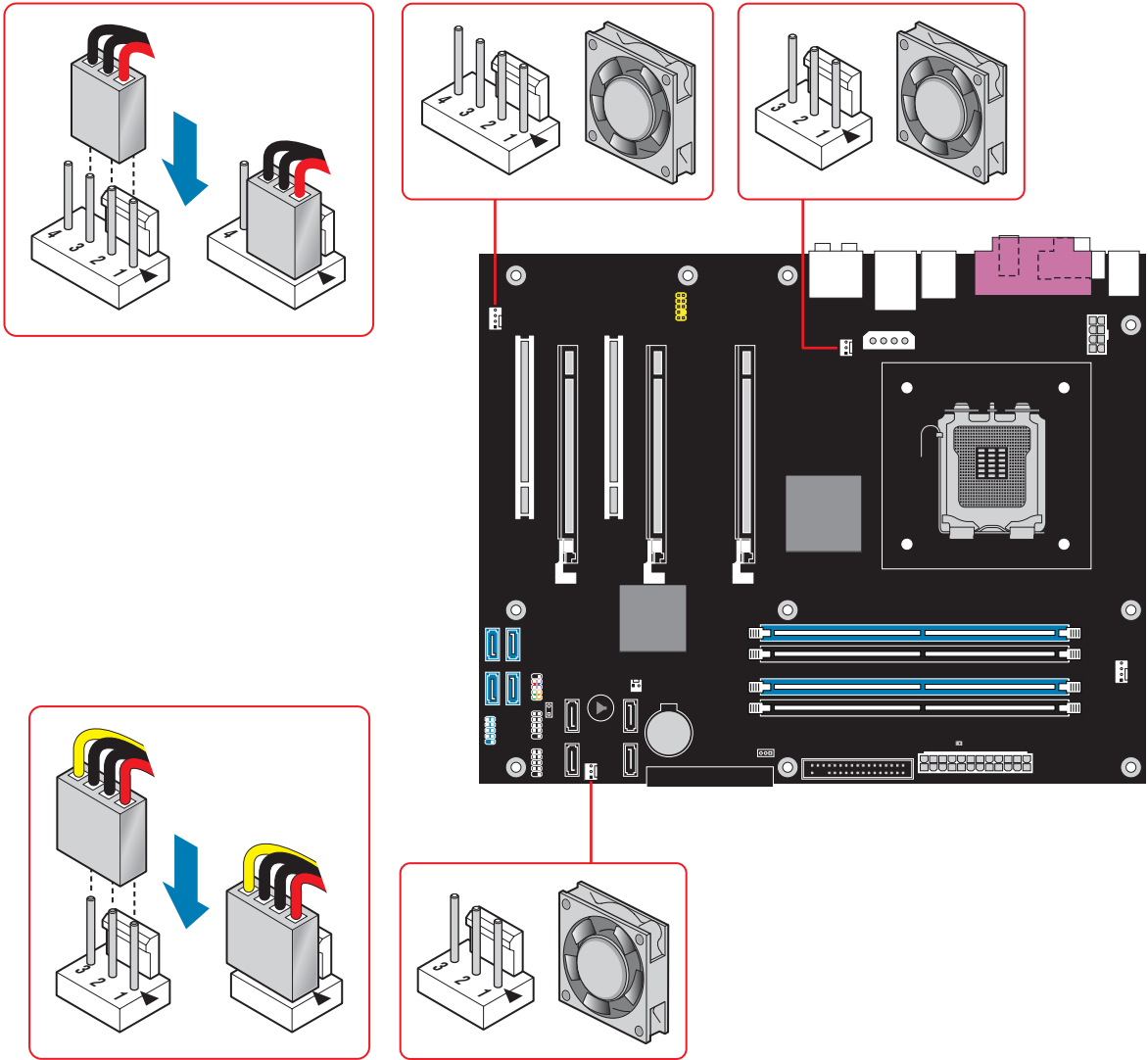
图 25. 风扇接头连接器位置
