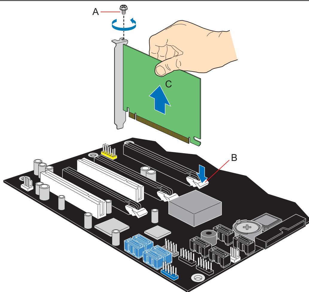
图 19. 拆卸 PCI Express x16 卡
