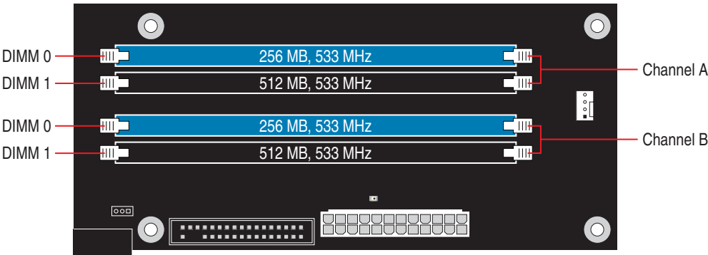
图 14. 双通道内存配置示例 2
