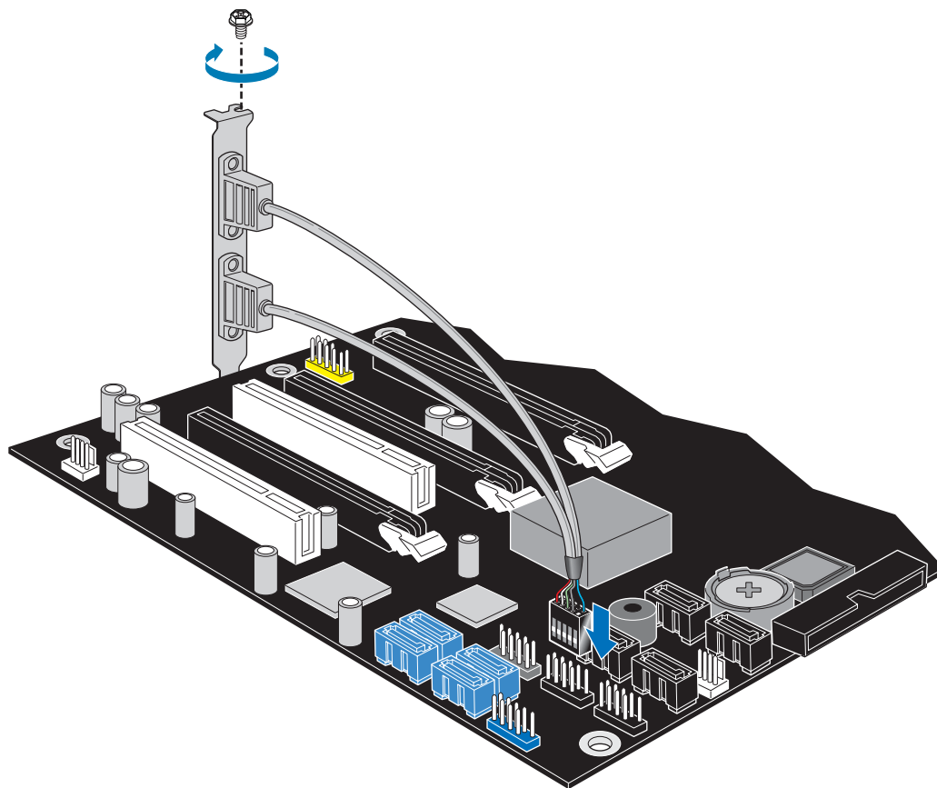
图 23. 连接背面板 USB 2.0 适配器
