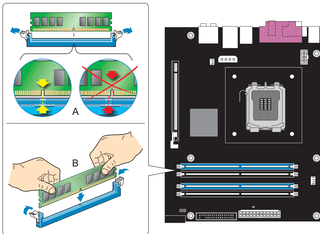
图 17. 安装 DIMM
