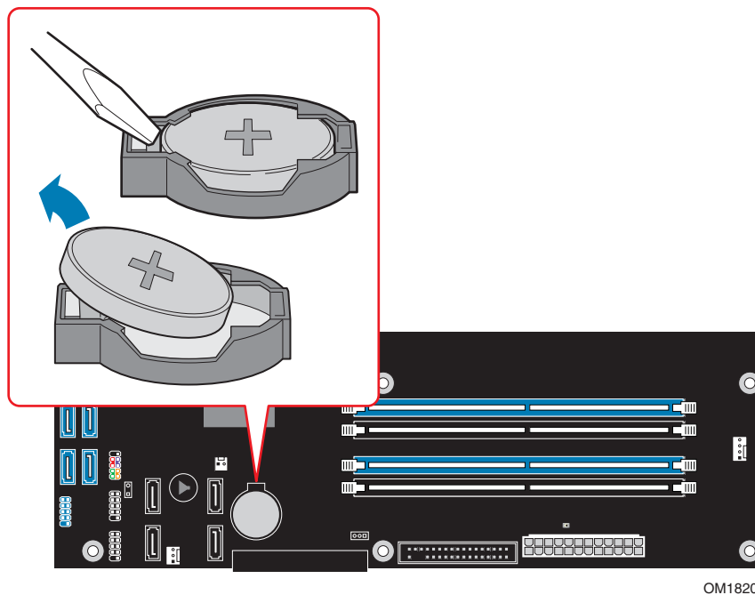
图 31. 拆卸电池
